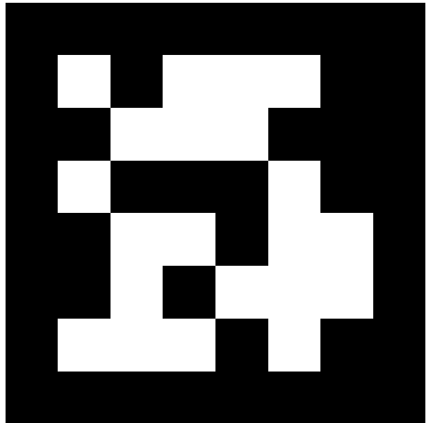
april.tag.Tag36h11, id = 139
