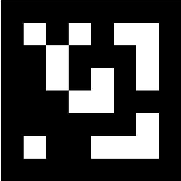
april.tag.Tag36h11, id = 212
