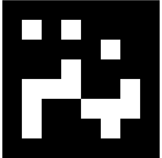
april.tag.Tag36h11, id = 125
