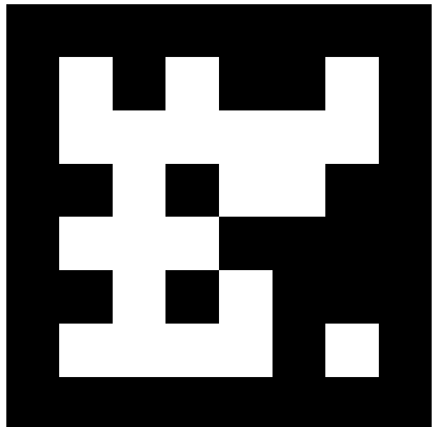
april.tag.Tag36h11, id = 463
