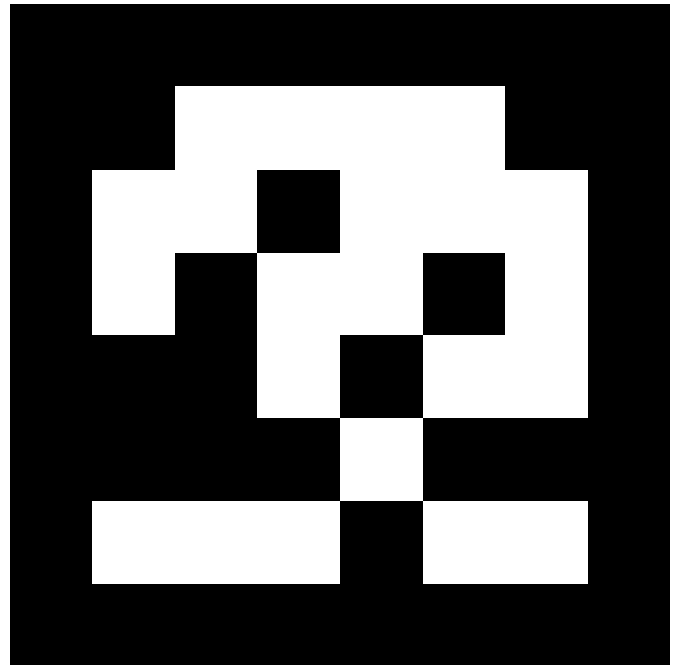
april.tag.Tag36h11, id = 195
