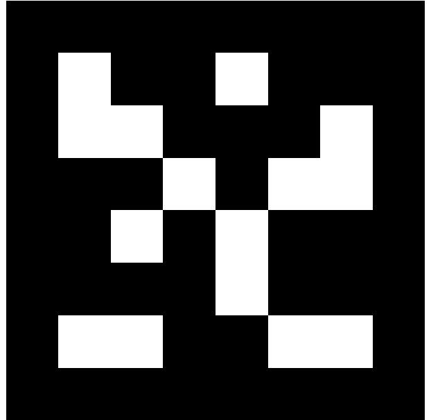
april.tag.Tag36h11, id = 489
