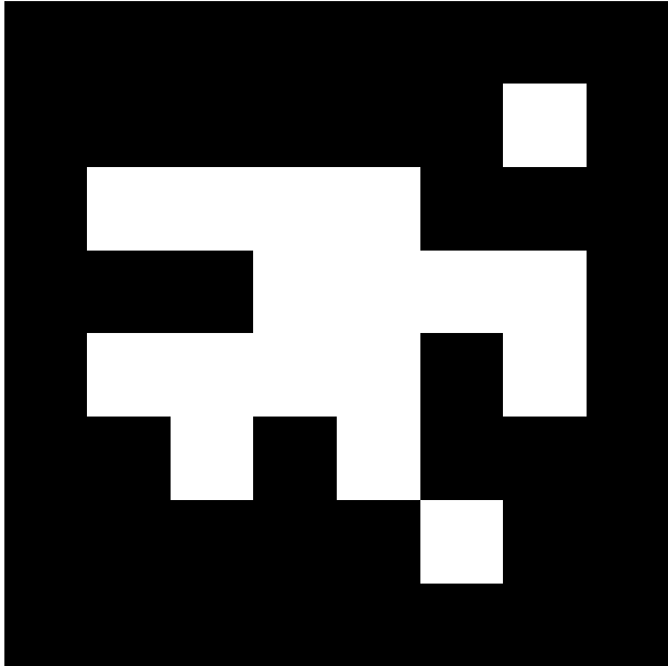
april.tag.Tag36h11, id = 176
