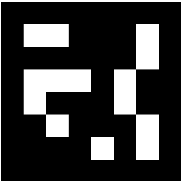
april.tag.Tag36h11, id = 54
