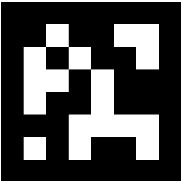
april.tag.Tag36h11, id = 14
