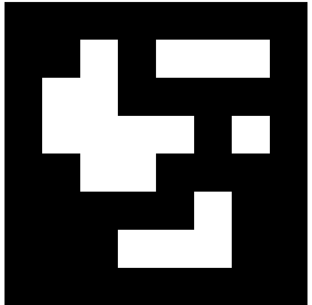
april.tag.Tag36h11, id = 503
