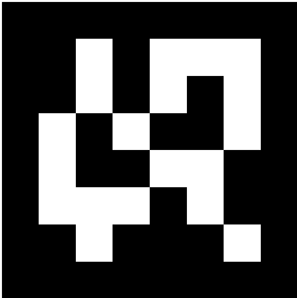
april.tag.Tag36h11, id = 202
