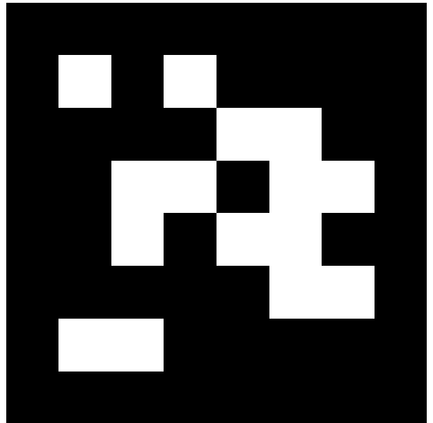
april.tag.Tag36h11, id = 291
