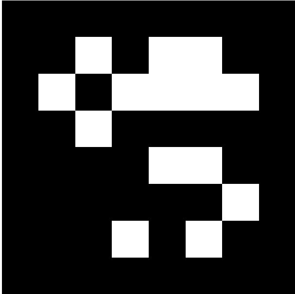
april.tag.Tag36h11, id = 80
