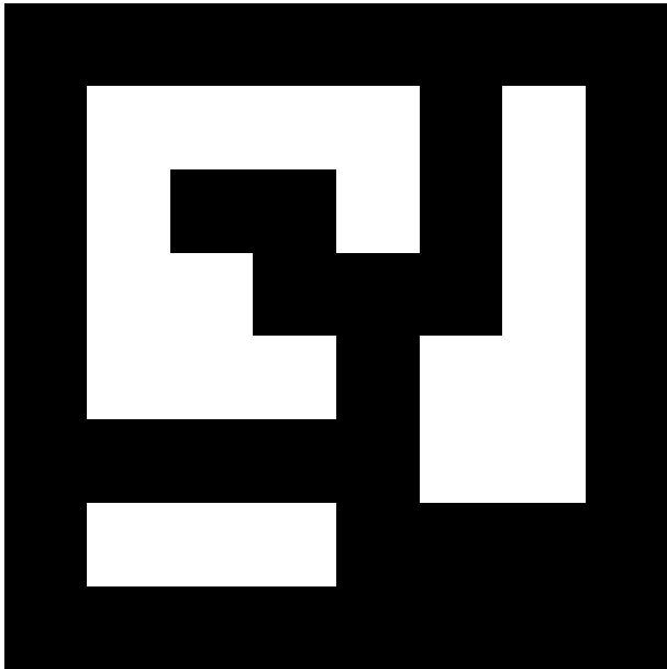
april.tag.Tag36h11, id = 424
