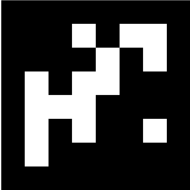
april.tag.Tag36h11, id = 452
