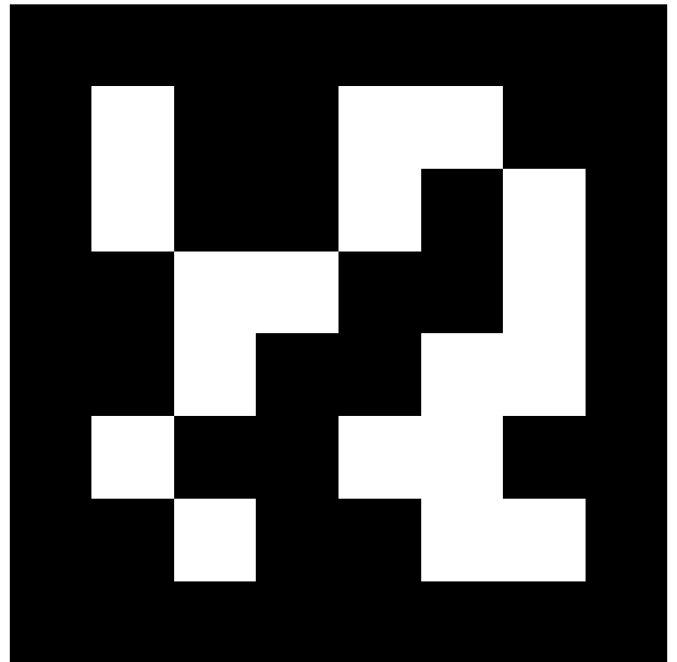
april.tag.Tag36h11, id = 103
