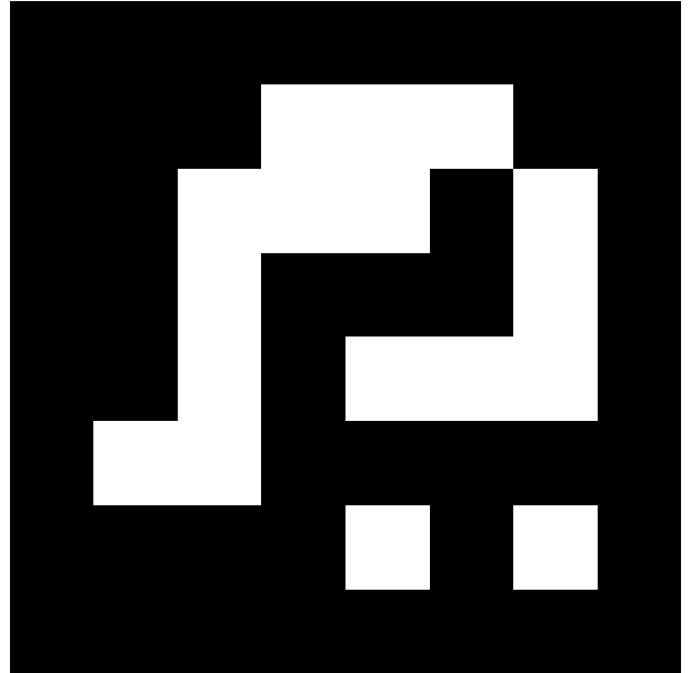
april.tag.Tag36h11, id = 397
