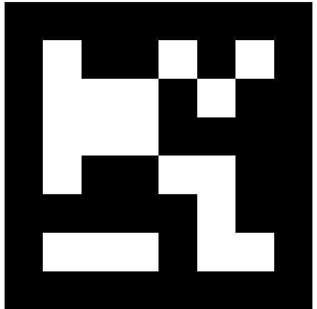
april.tag.Tag36h11, id = 531
