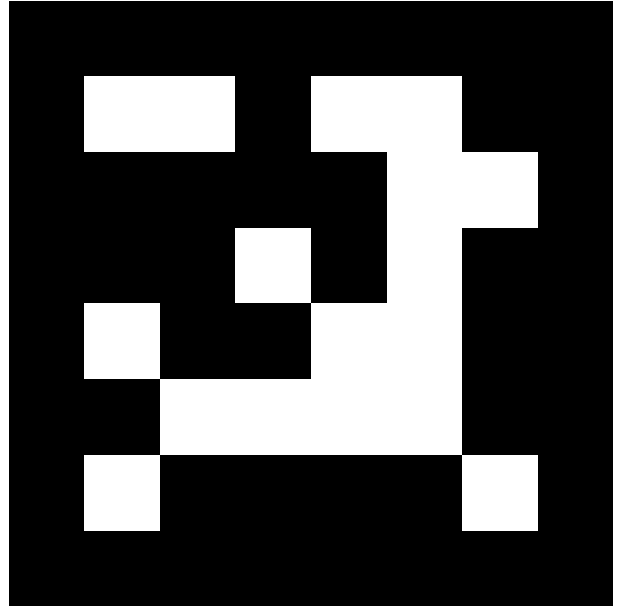
april.tag.Tag36h11, id = 133
