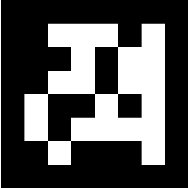
april.tag.Tag36h11, id = 332
