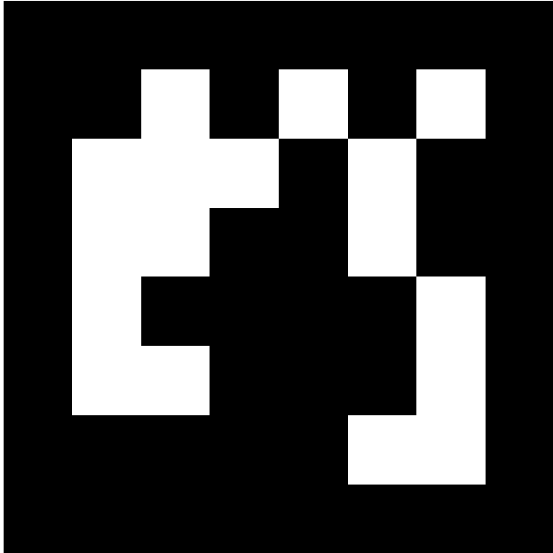
april.tag.Tag36h11, id = 408
