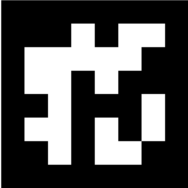
april.tag.Tag36h11, id = 508
