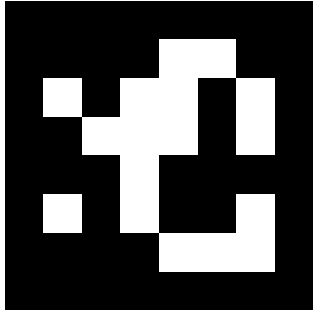
april.tag.Tag36h11, id = 245
