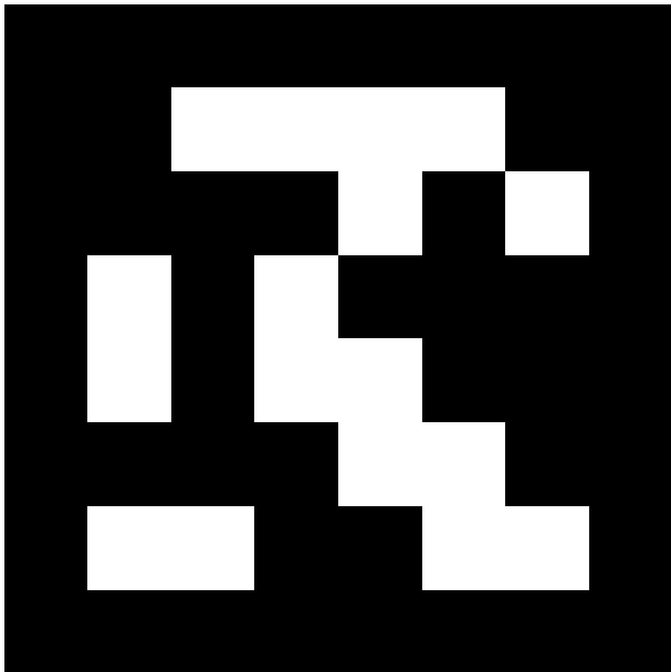
april.tag.Tag36h11, id = 410
