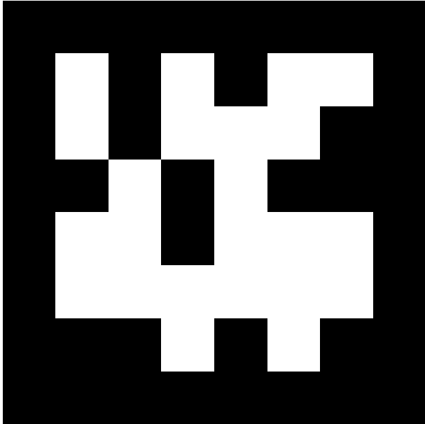
april.tag.Tag36h11, id = 168
