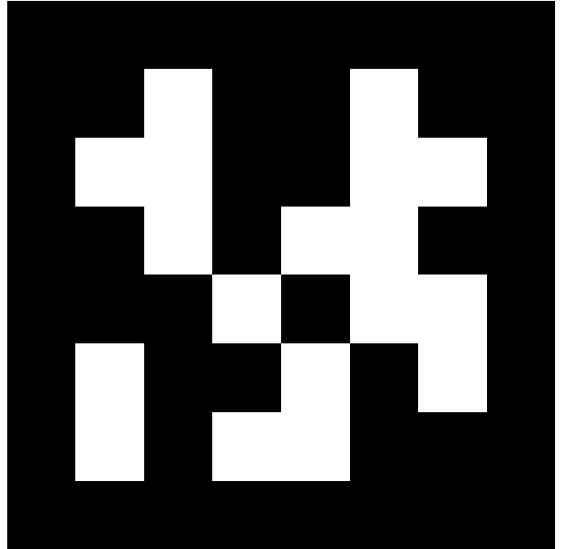
april.tag.Tag36h11, id = 137
