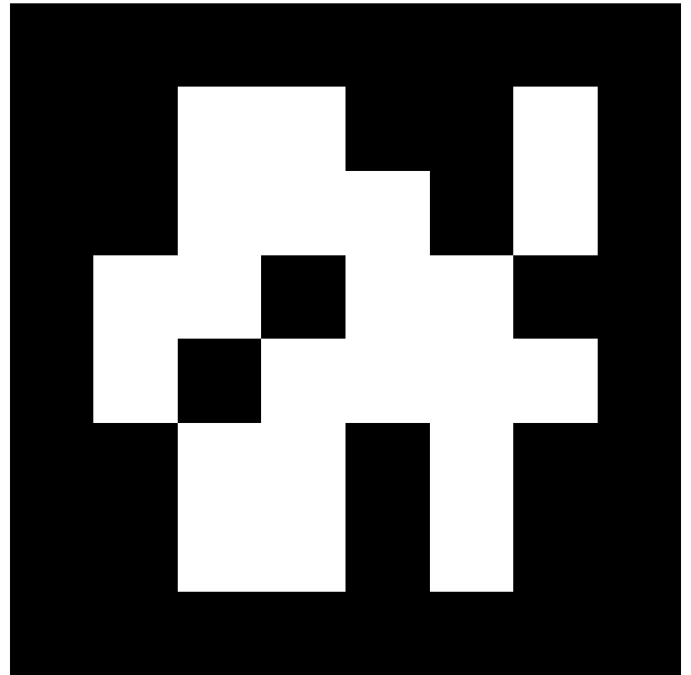
april.tag.Tag36h11, id = 425
