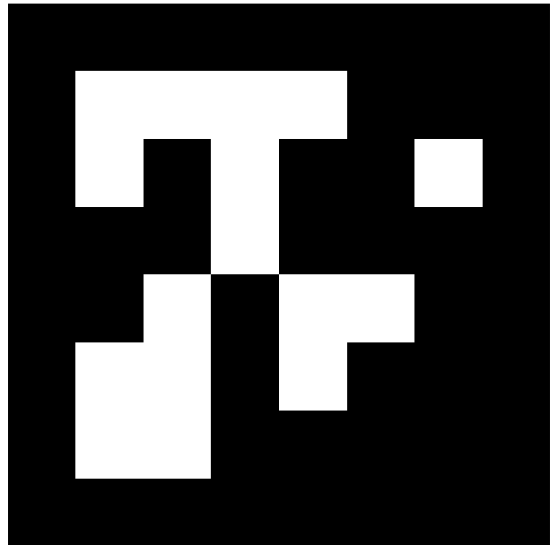
april.tag.Tag36h11, id = 247
