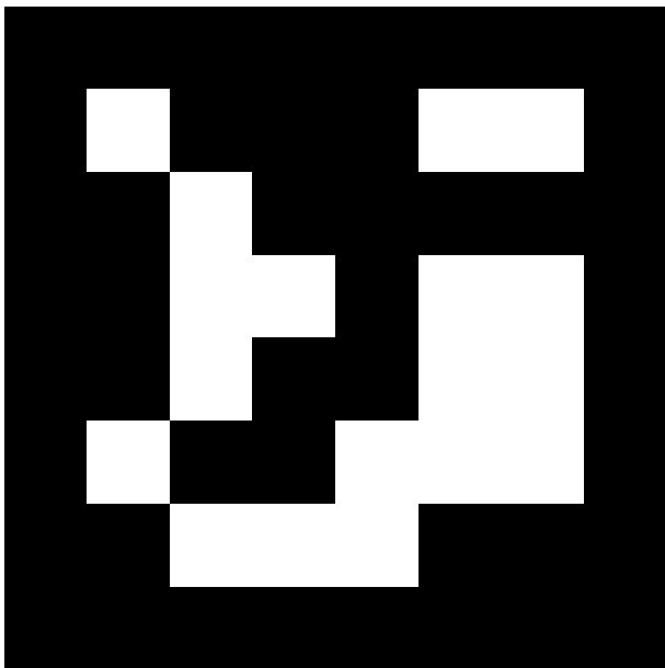
april.tag.Tag36h11, id = 38
