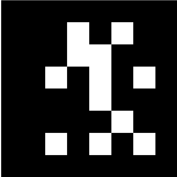
april.tag.Tag36h11, id = 396
