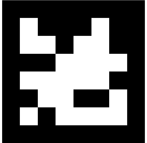
april.tag.Tag36h11, id = 309
