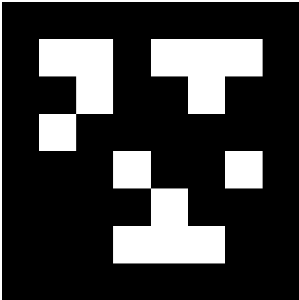
april.tag.Tag36h11, id = 2
