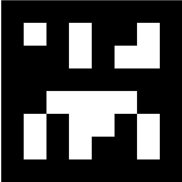
april.tag.Tag36h11, id = 412
