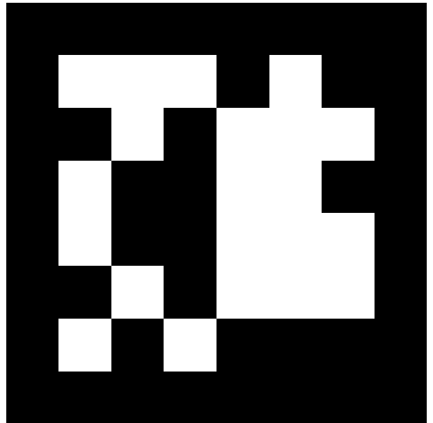
april.tag.Tag36h11, id = 383
