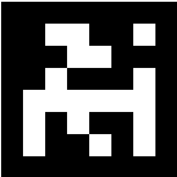
april.tag.Tag36h11, id = 34
