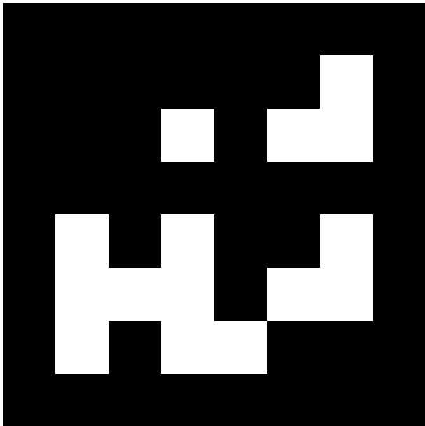
april.tag.Tag36h11, id = 510
