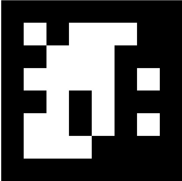
april.tag.Tag36h11, id = 252
