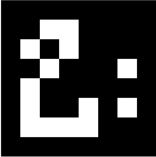
april.tag.Tag36h11, id = 180
